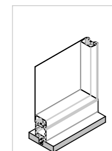
Monofacciale Motorizzato
